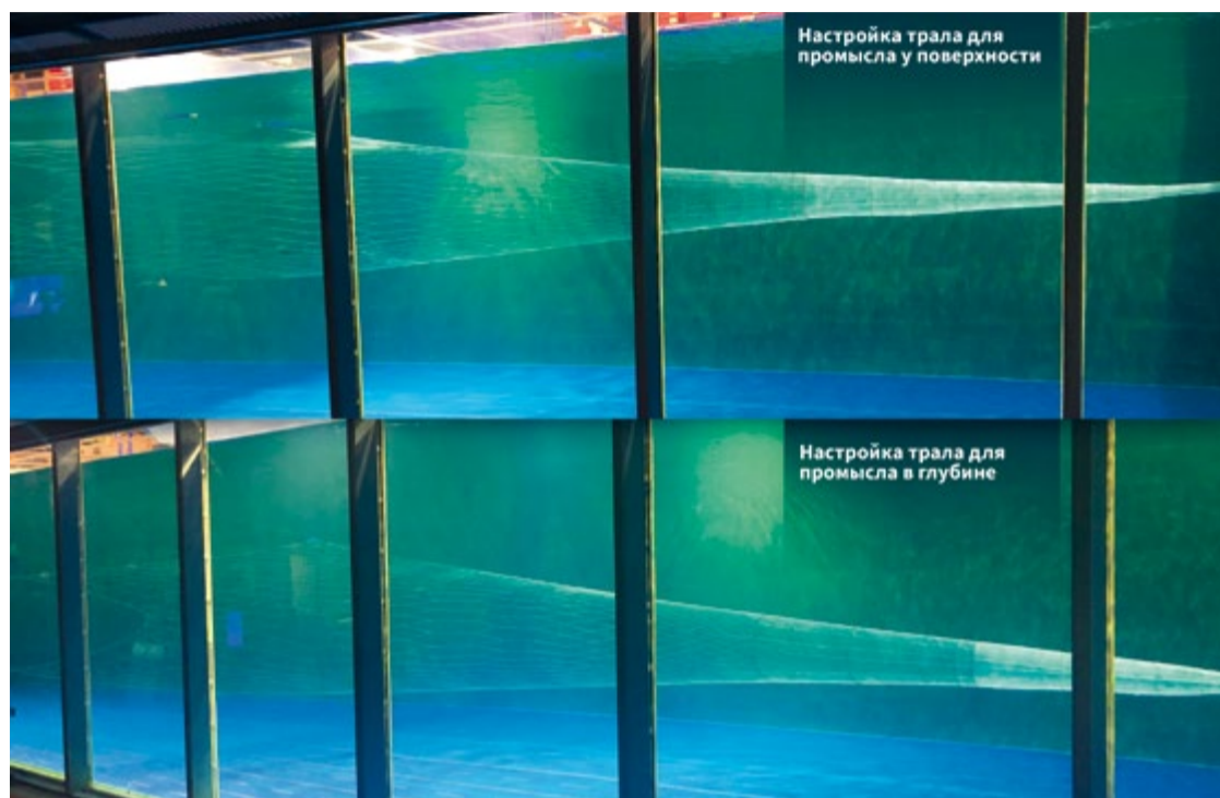
Новый трал «Атлантика-1790» – настройка для различных условий промысла
