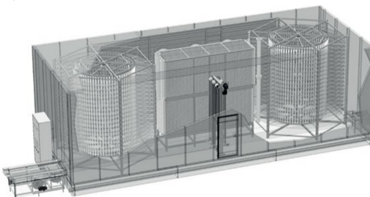
Спиральная морозильная установка
